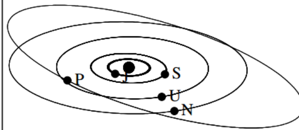
Störmer-Verlet, h = 200
